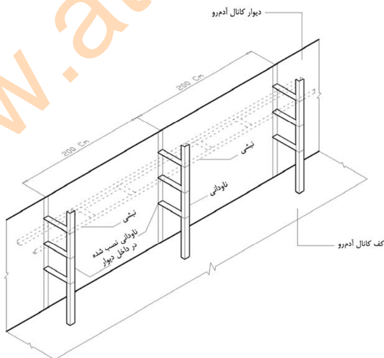
شکل ۸-۳: جزئیات تپانجه‌بندی اسکلت‌بندی نصب کابل در داخل کانال‌های آدمرو
