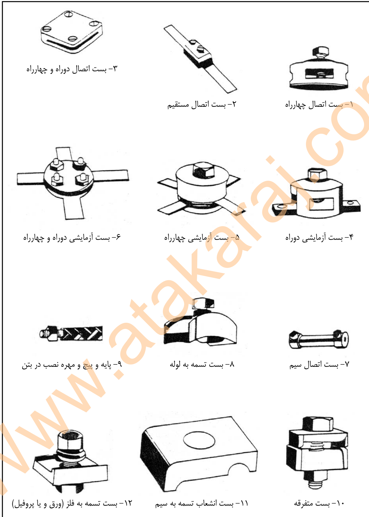
شکل ۱۴-۱۱: اتصالات و وسایل مختلف تسمه‌کشی
