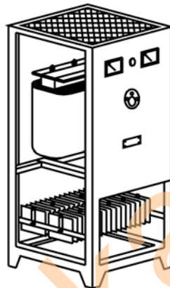
شکل ۲-۱۲: نمونه مجموعه یکسوساز شامل پشته‌های یکسوکننده، ترانسفورماتور و لوازم فرعی
