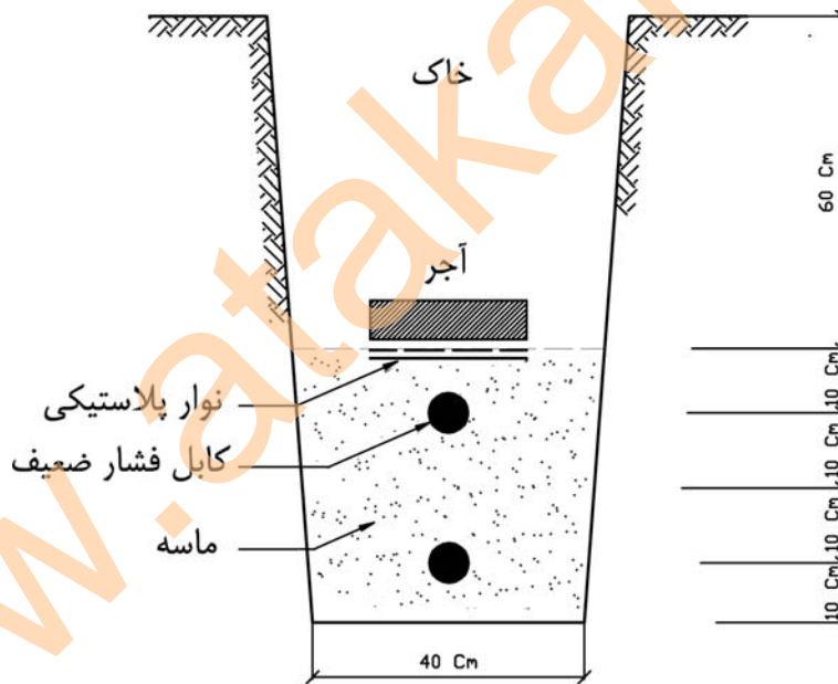
جزییات کانال خاکی تیب برای نصب کابل فشار ضعیف در دو ردیف افقی
